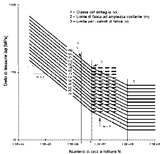
Figura C4.2.21 - Curve S-N per dettagliolementi soggetti a tensioni normali
